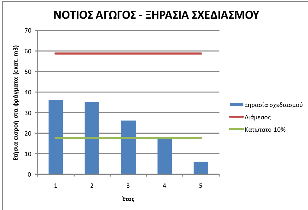
Σχήμα 4-2: Σύγκριση Αθροιστικής Κατανομής Ιστορικού και Συνθετικών Δειγμάτων Ετήσιου όγκου εισροής στα φράγματα για την πενταετή περίοδο ξηρασίας σχεδιασμού.
