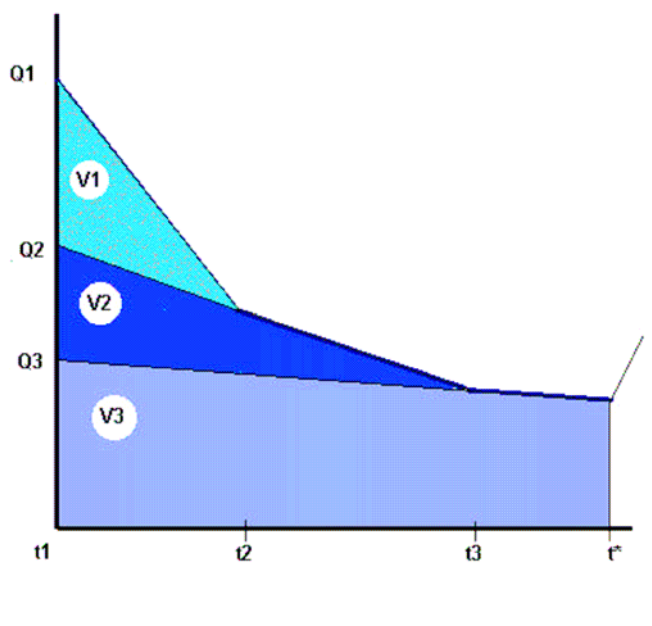
Σχήμα 8-4: Διαφορετικοί συντελεστές στείρευσης και αντίστοιχοι όγκοι αποθεμάτων από διαφορετικούς μηχανισμούς
