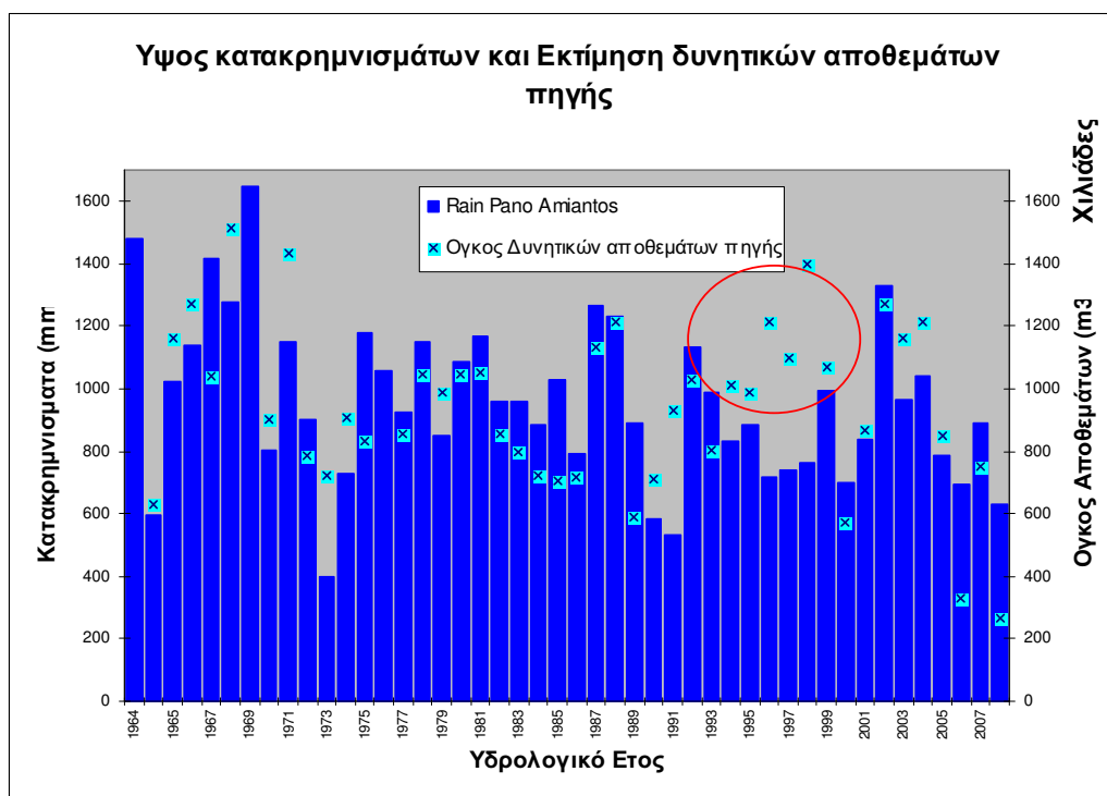
Σχήμα 8-7: Εκτίμηση δυνητικών αποθεμάτων πηγής s9-6-3-50 (ARKOLAKHANIA) και ετήσιο ύψος κατακρημισμάτων ανάντη της πηγής σταθμού (Πάνω Αμίαντος). Υπογραμμίζεται χρονική περιοχή με αμφίβολα αποτελέσματα
