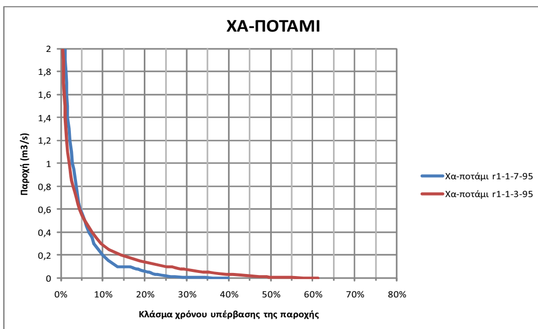
Σχήμα 8-12: Σχέση παροχής-διάρκειας
