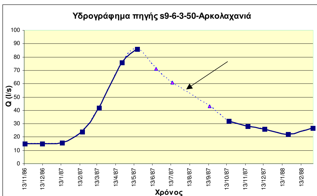
Σχήμα 8-5: Επιλογή κλάδου υδρογραφήματος (στικτή γραμμή) για εκτίμηση «α» και S (δυνητικών αποθεμάτων)
