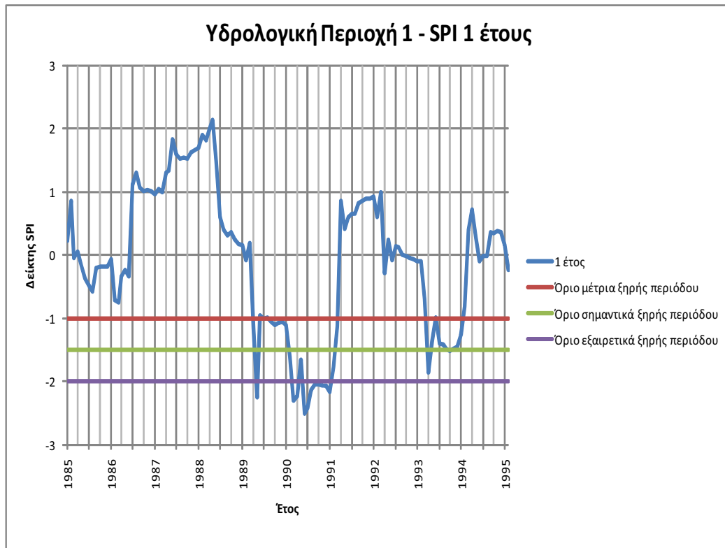
Σχήμα 2-2: Δείκτης SPI 12 μηνών για Υδρολογική Περιοχή 1 (Υδρολογική Περίοδος 1985-1995)
