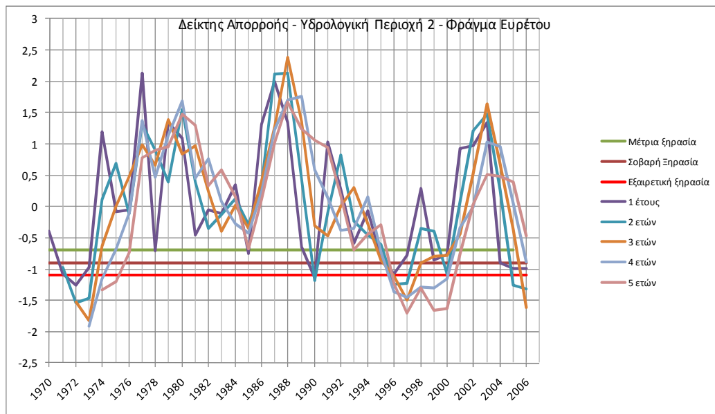
Σχήμα 2-11: Σύγκριση Δεικτών Απορροής Υδρολογικής Περιοχής 2
