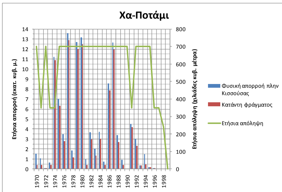
Σχήμα 8-15: Προσομοίωση ισοζυγίου φράγματος
