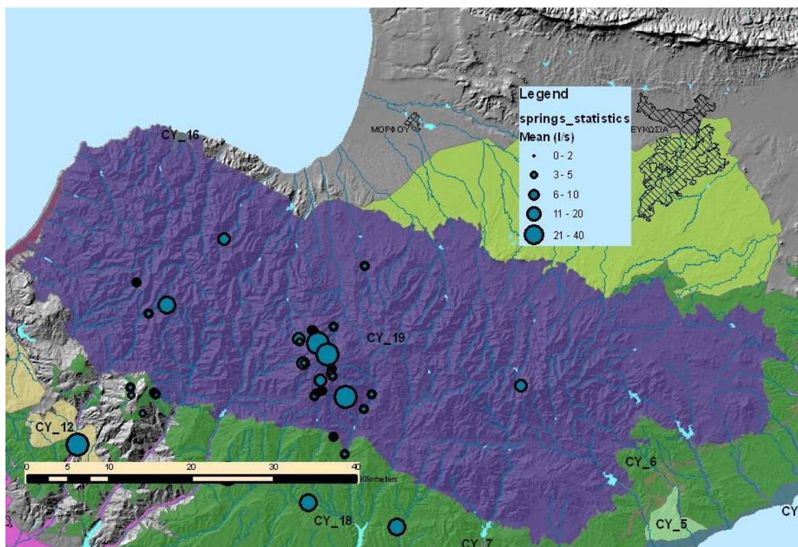
Σχήμα 8-2: Πηγαίες αναβλύσεις και μέσες τιμές παροχών(l/s).
