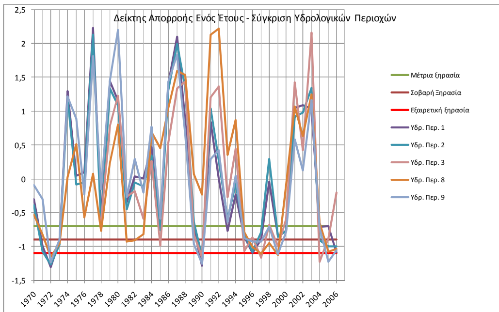
Σχήμα 2-15: Σύγκριση Δείκτη Απορροχής Ενός (1) Έτους Συνόλου Υδρολογικών Περιοχών
