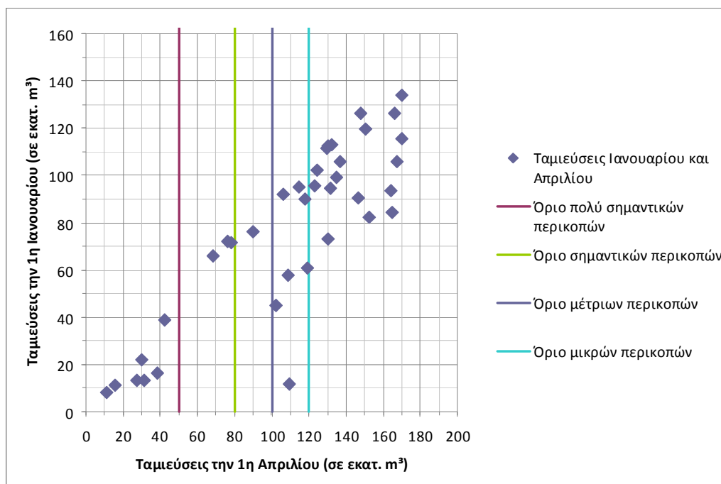
Σχήμα 4-4: Συσχέτιση όγκου ταμίευσης 1 ης Ιανουαρίου και 1 ης Απριλίου και Προτεινόμενα Όρια Περικοπών
