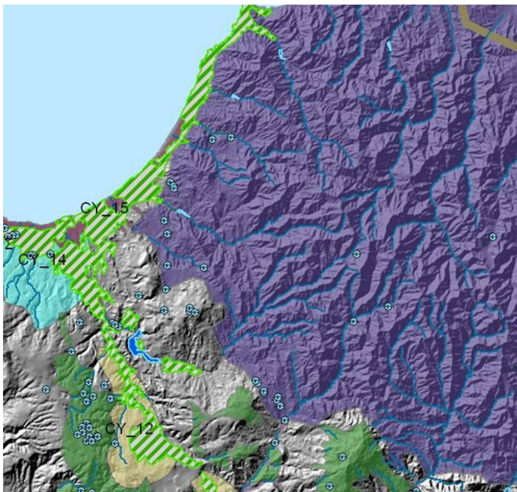
Σχήμα 7-2: Υδρευτικές γεωτρήσεις (κυανό) στην περιοχή έργου Χρυσοχούς
