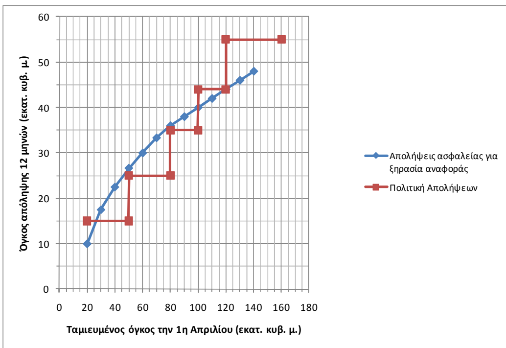
Σχήμα 4-2: Πολιτική Απολήψεων και Εκτιμήσεις Απολήψεων Ασφαλείας
