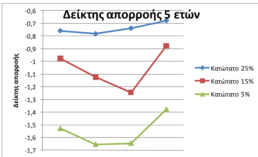
Σχήμα 2-9: Συσχέτιση Δείκτη Απορροής με Σπανιότητα Εμφάνισης (5 ετών)
