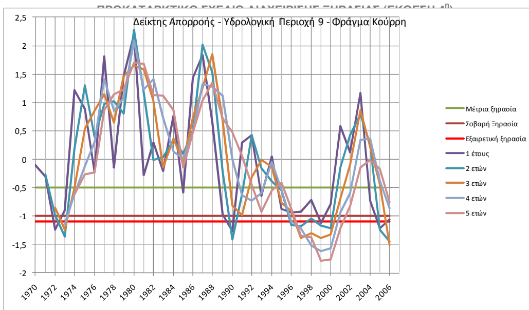
Σχήμα 2-14: Σύγκριση Δεικτών Απορροχής Υδρολογικής Περιοχής 9
