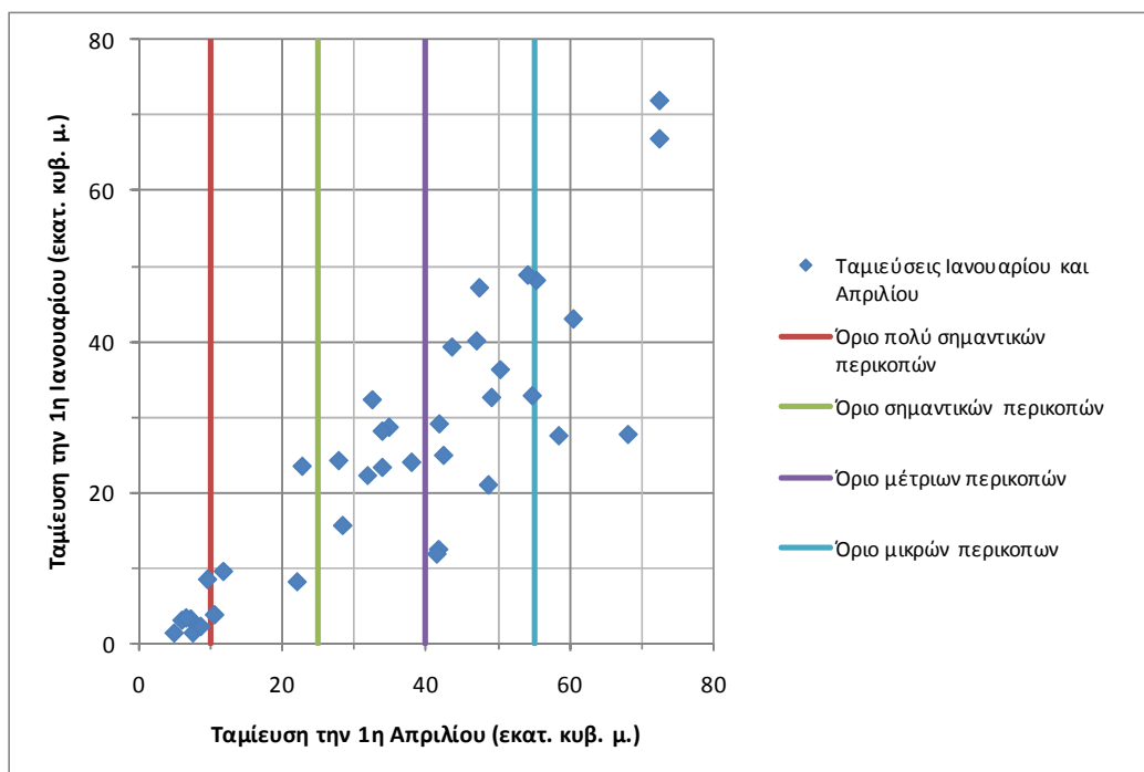
Σχήμα 6-4: Συσχέτιση όγκου ταμίευσης 1 ης Ιανουαρίου και 1 ης Απριλίου και Προτεινόμενα Όρια Περικοπών
