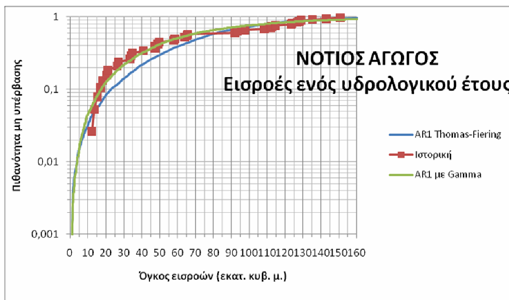
Σχήμα 4-1: Σύγκριση Αθροιστικής Κατανομής Ιστορικού και Συνθετικών Δειγμάτων
