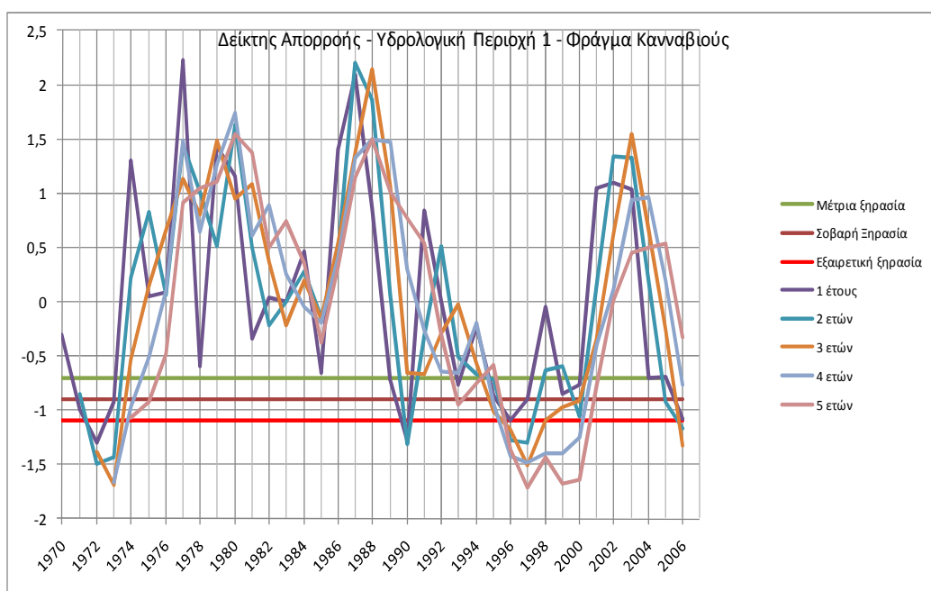
Σχήμα 2-10: Σύγκριση Δεικτών Απορροής Υδρολογικής Περιοχής 1
