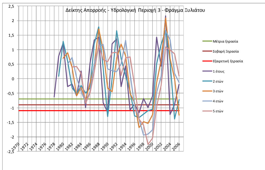
Σχήμα 2-12: Σύγκριση Δεικτών Απορροής Υδρολογικής Περιοχής 3
