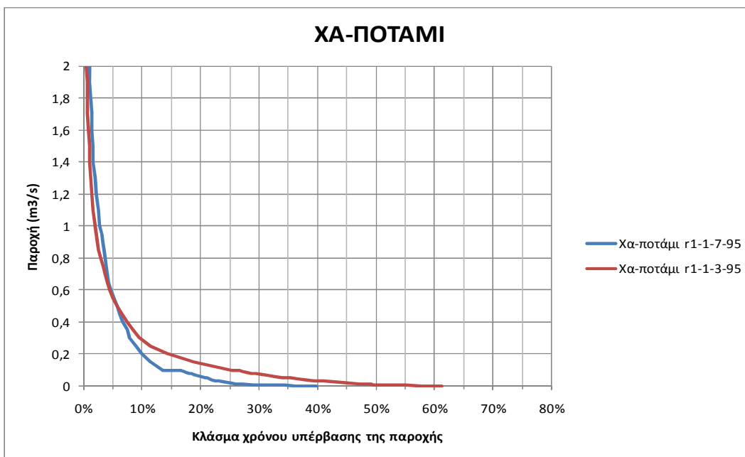
Σχήμα 8-12: Σχέση παροχής-διάρκειας
