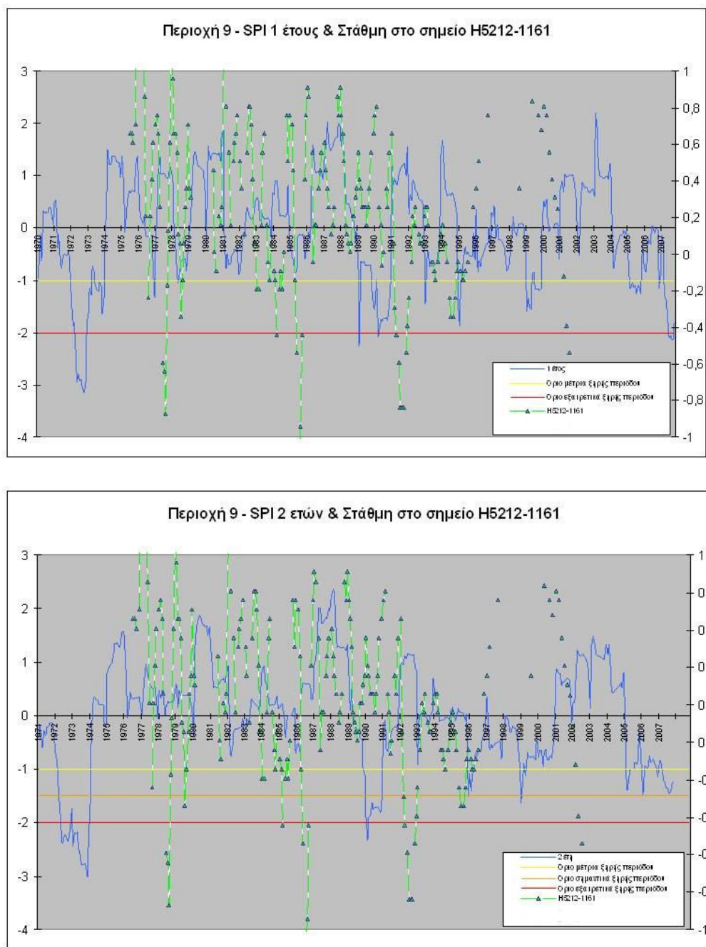
Σχήμα 2-22: Στάθμη Υπογείου Νερού και Δείκτης Ξηρασίας (SPI) – Ακρωτήρι
