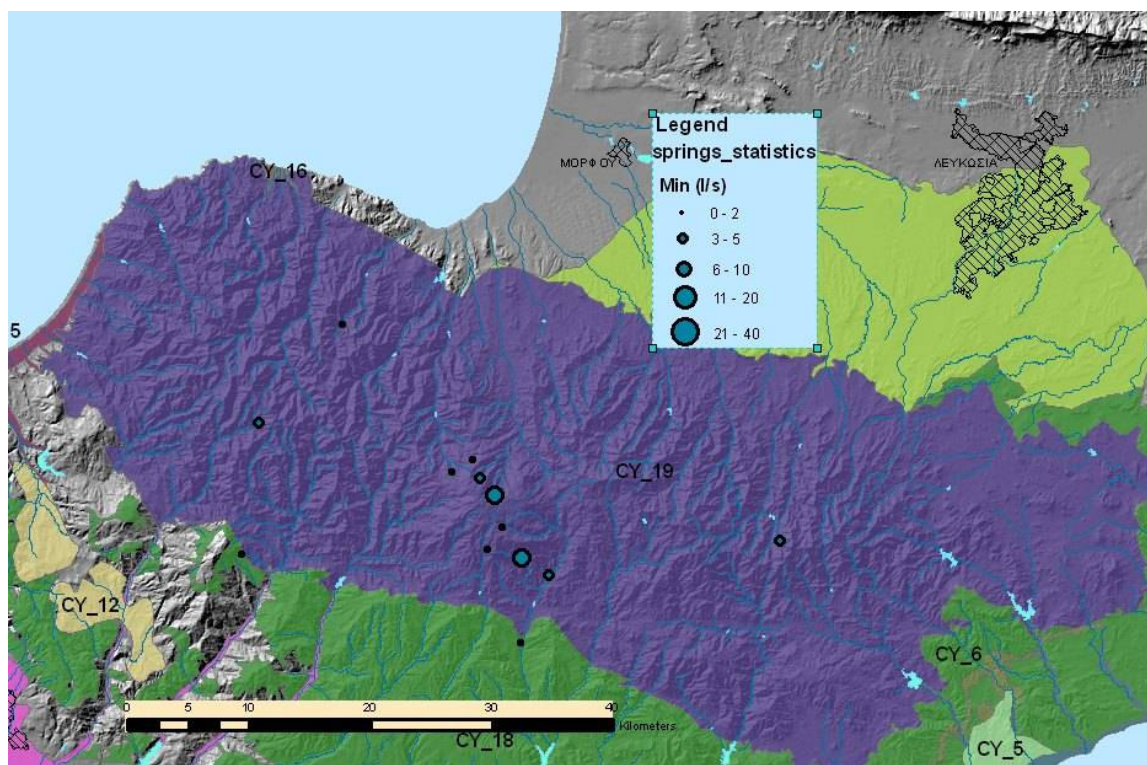
Σχήμα 8-8: Πηγαίες αναβλύσεις και ελάχιστες τιμές παροχών(l/s).
