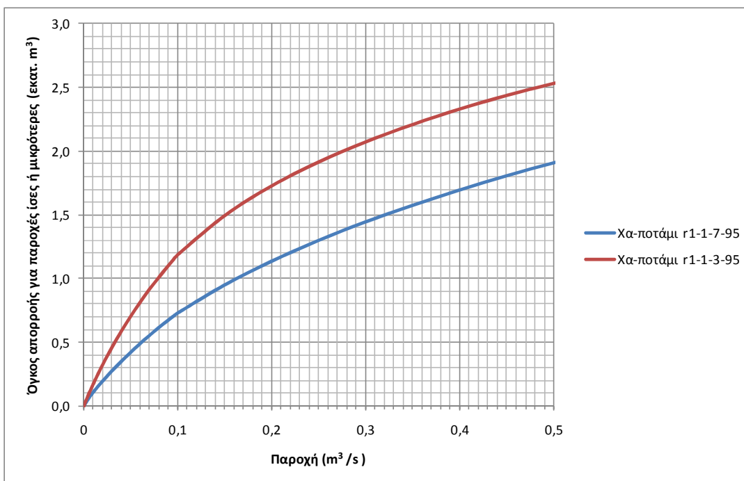
Σχήμα 8-14: Χα-ποτάμι, σχέση ογκο απορροής-παροχής
