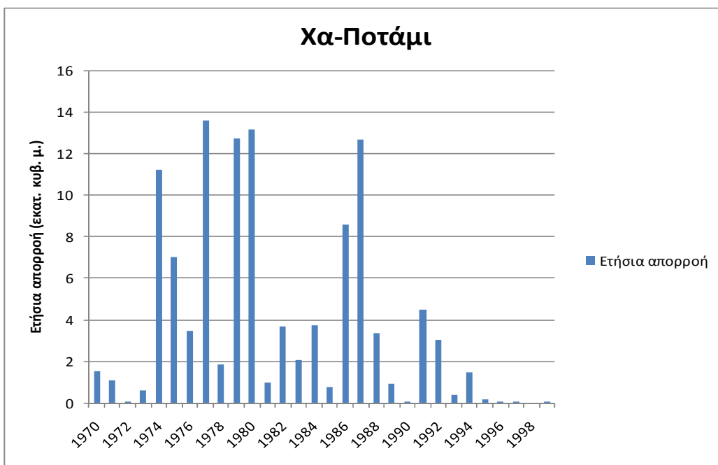
Σχήμα 8-11: Ετήσιος όγκος απορροής στο Χα-ποτάμι, στα κατάντη της υδροληψίας Κισσούσας και ανάντη της υδροληψίας Πισσουριού-Αλέκτορα προ της λειτουργίας της εκτροπής προς Κούρρη
