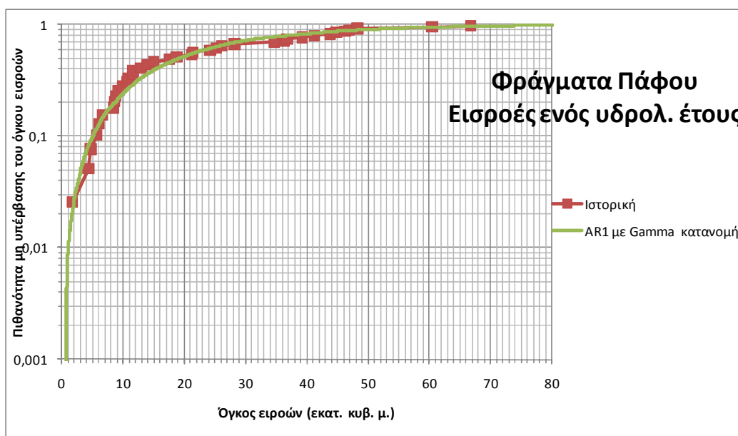
Σχήμα 6-1: Σύγκριση Αθροιστικής Κατανομής Ιστορικού και Συνθετικών Δειγμάτων
