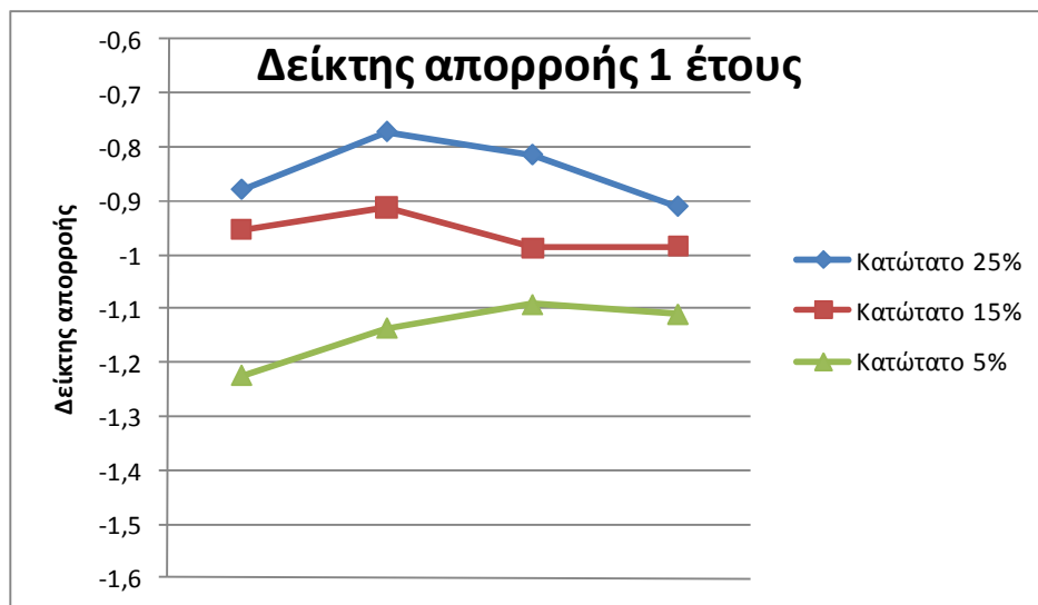
Σχήμα 2-5: Συσχέτιση Δείκτη Απορροής με Σπανιότητα Εμφάνισης (1 έτους)
