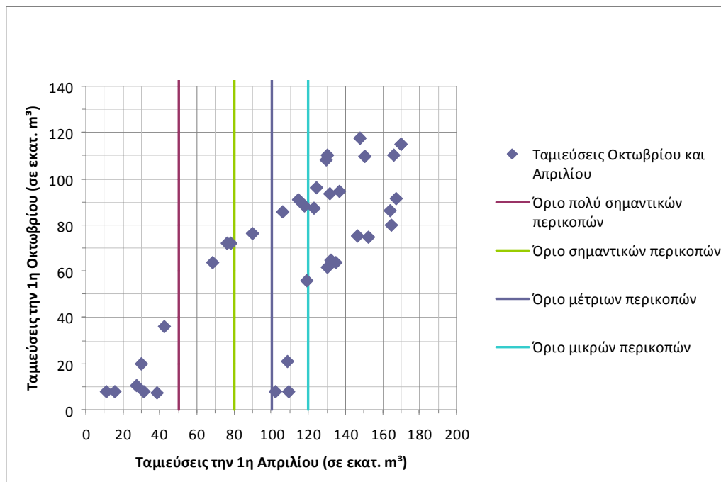
Σχήμα 4-3: Συσχέτιση όγκου ταμίευσης 1 ης Οκτωβρίου και 1 ης Απριλίου και Προτεινόμενα Όρια Περικοπών
