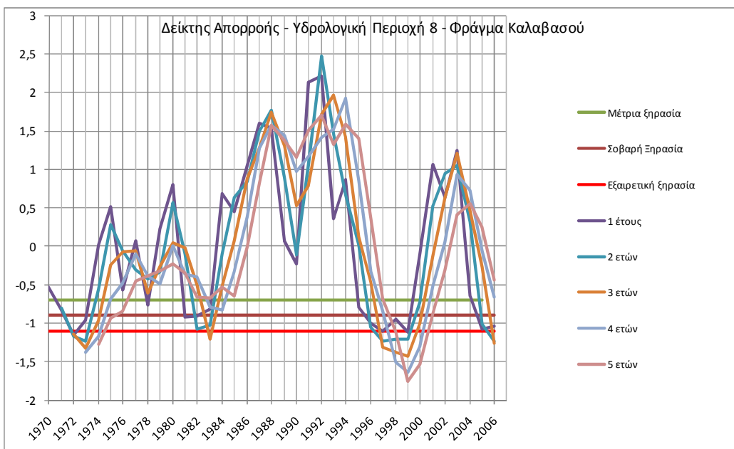
Σχήμα 2-13: Σύγκριση Δεικτών Απορροής Υδρολογικής Περιοχής 8
