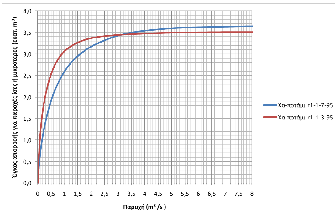
Σχήμα 8-13: Χα-ποτάμι, σχέση όγκου απορροής-παροχής
